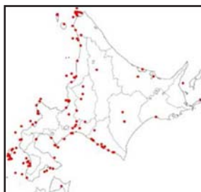
第1図 北海道の竜巻分布図 (1961～2015年)
