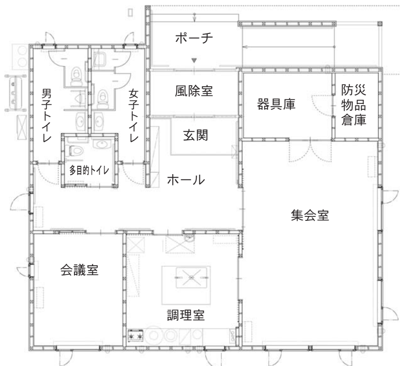
【千栄会館平面図】
